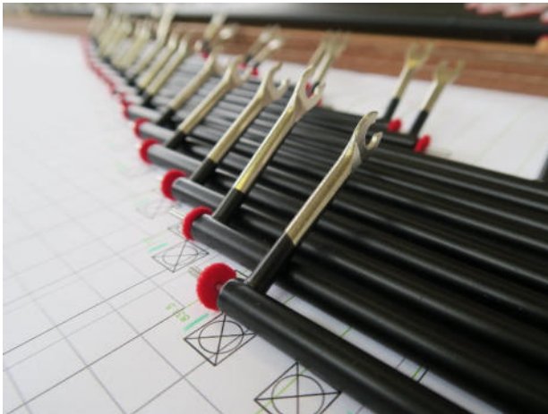
1.1 Punktgeschweisste Trakturwellen
